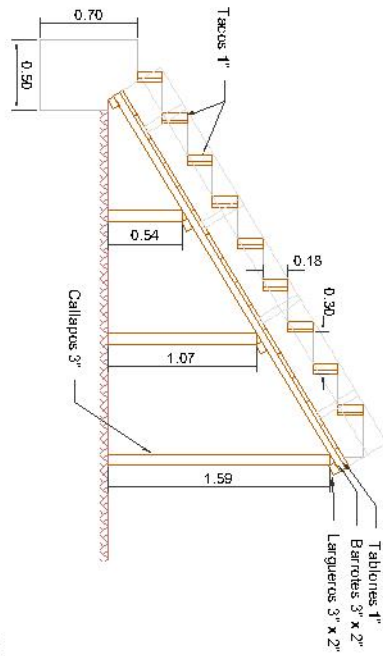
Encofrado Lateral Escalera Esc. 1:50
