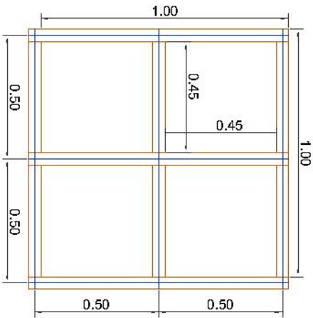
Estructura de Madera Esc. 1:20
