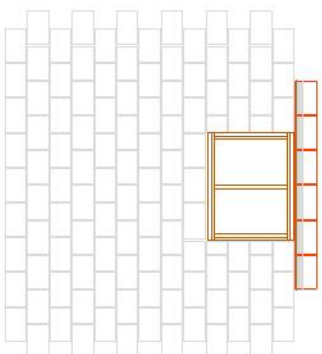
Dintel para Ventana Esc. 1:30
