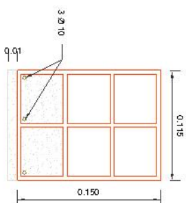
Sección Dintel Esc. 1:35
