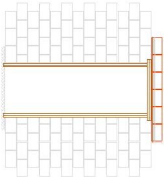
Dintel para Puerta Esc. 1:30
