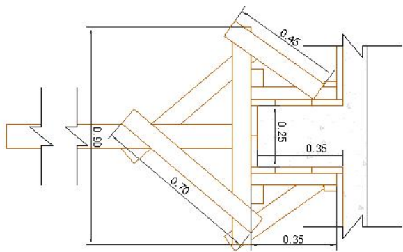
Encofrado Viga Esc. 1:20
