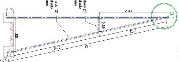
Elevación Lateral: Estructura Esc. 1:50
