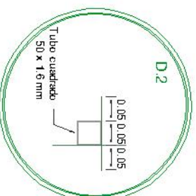
Planta: Anclaje Parantes Esc. 1:10
