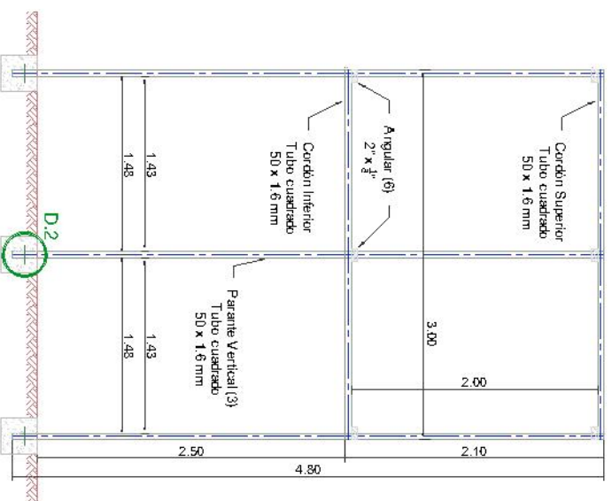
Elevación Frontal: Estructura Esc. 1:50
