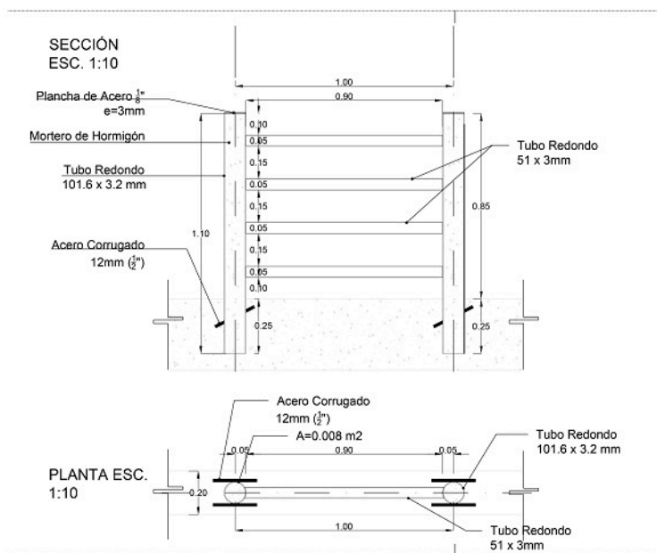
BARANDA DE PROTECCION EN VIADUCTOS CON TUBO REDONDO 101,6 X 3,2 mm RELLENO CON H° S° DOSIF 1:2:4
