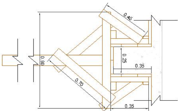
Encofrado Viga Esc. 1:20
