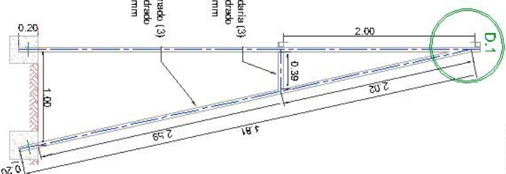
Planta: Anclaje Parantes
