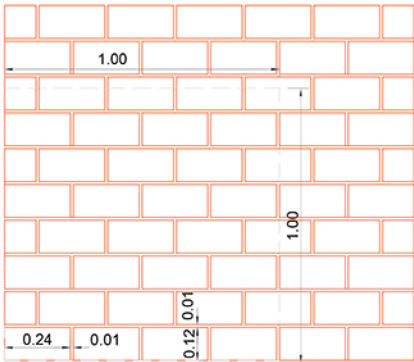
Muro de Ladrillo Esc. 1:20
