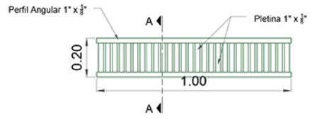
Sumidero para Gradería Esc. 1:20
