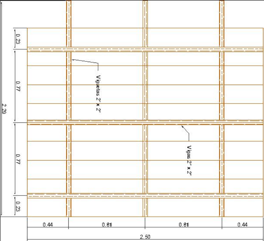
Encofrado Losa Esc: 1:25
