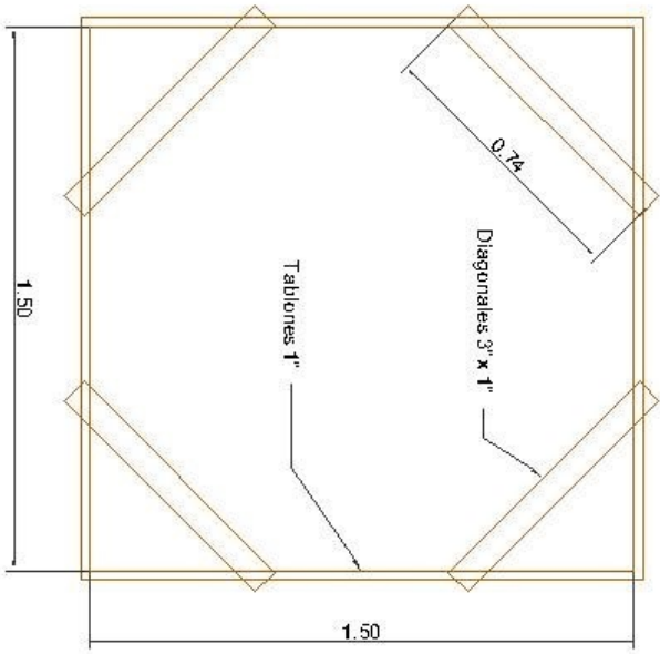
Puntales
