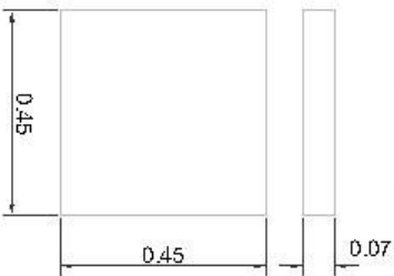
Tapa Cámara
