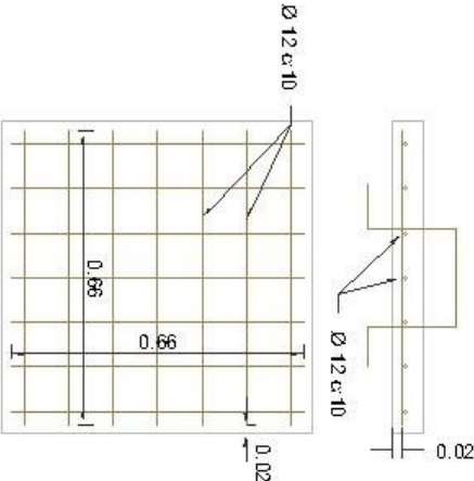
Armadura tapa Esc. 1:20
