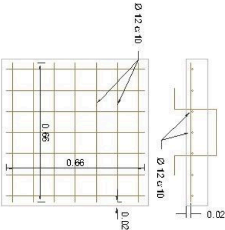
Armadura tapa Esc. 1:20
