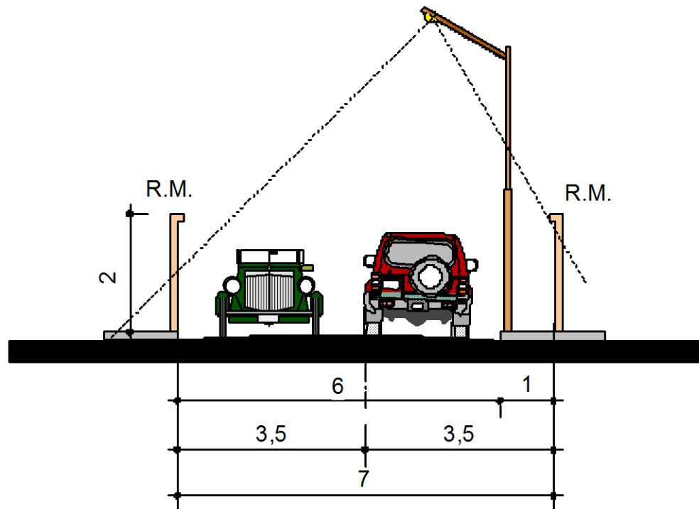
Perfil de Vía de 7.00 mts.
