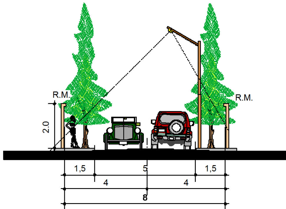
Perfil de Vía de 8.00 mts.
