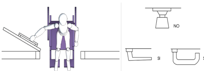
CARACTERÍSTICAS DE MANILLAS
