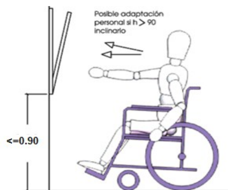
ESPEJO USUARIO EN SILLA DE RUEDAS
