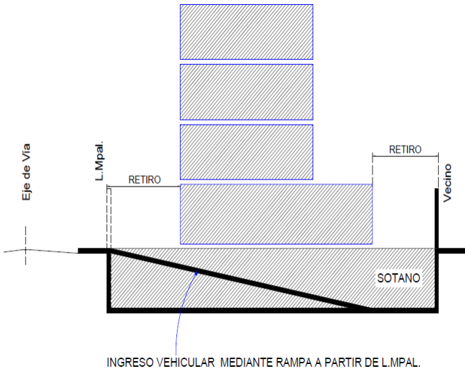
Esquema de Ingreso a Sótano para Patrones 4, 4CP, 5, 5Z, 6, 6Z.
