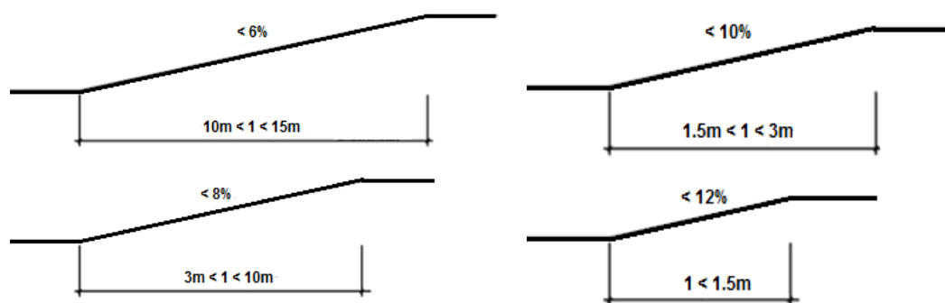
PENDIENTE LONGITUDINAL EN FUNCIÓN A LA EXTENSIÓN
