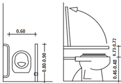
BARRAS DE APOYO: COLOCACIÓN EN INODOROS
