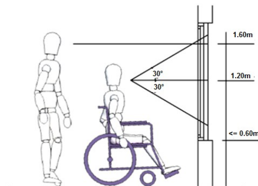
PLANO HORIZONTAL - ALTURAS AL NIVEL DEL OJO
